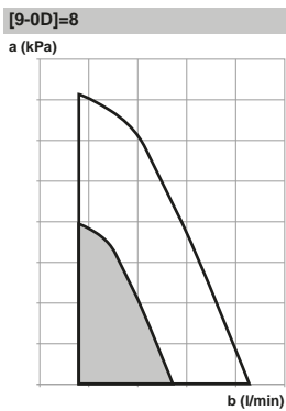
a Externer statischer Druck b Wasserdurchflussmenge
