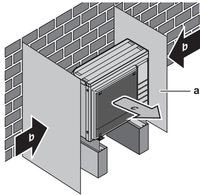
a Ablenkplatte b Vorherrschende Windrichtung c Luftauslass
